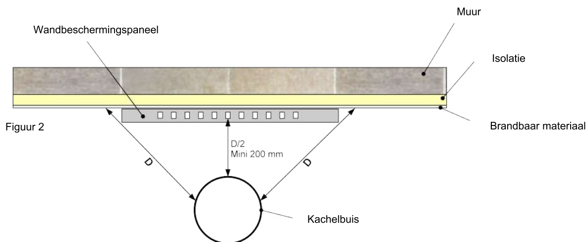
Figuur 2 - Regels voor het plaatsen van de kachel en het afvoer kanaal met betrekking tot brandbaar materiaal D = Afstand tot brandbare materialen zoals opgegeven door de fabrikant
