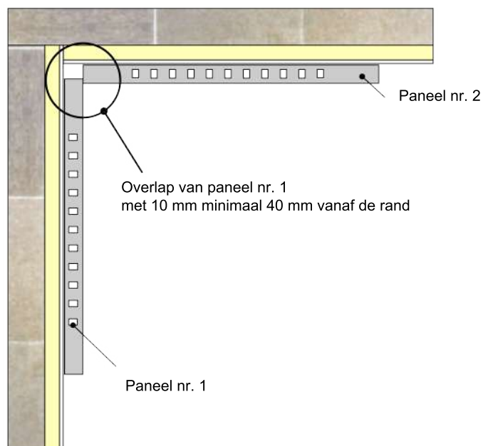
Figuur 3 - Het muurbeschermingspaneel installeren in een hoek met details over de montage van paneel nr. 1
